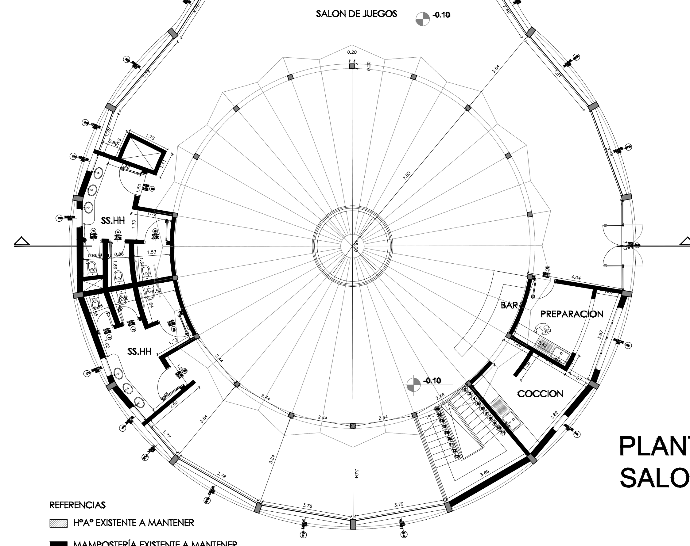
PLANTA BAJA S.U.M
